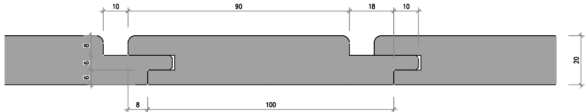
Nr. 2202-10-03 Sichtnutschalung gerade 20/100 mm, Nut 10 mm, Radius 3 mm
