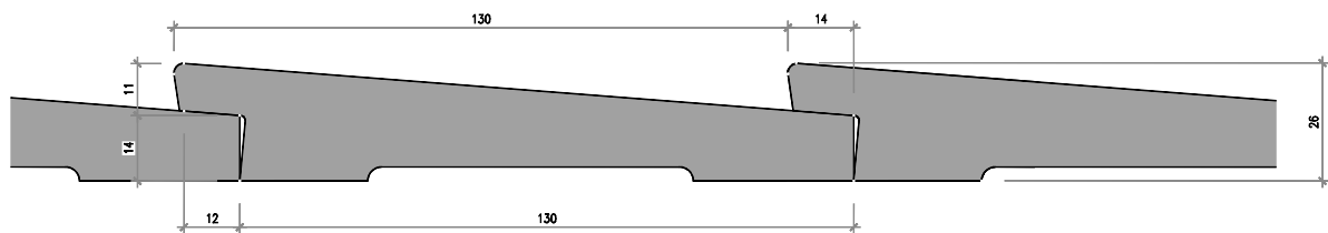
Nr. 7601-00-03 Stülpchalung Falz 14/26/130 mm, Rückseitig ausgekehlt
