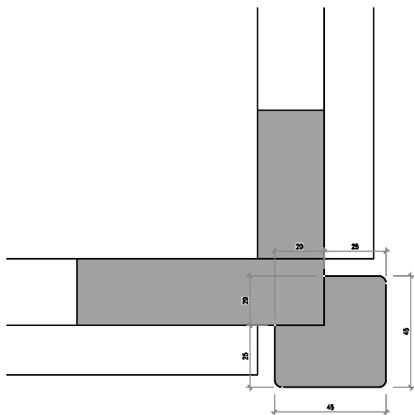
Nr. 82b01-3k-03 Fassadeneckprofil L 45/45 mm, 20/20 mm ausgekehrt, Radius 3 mm
