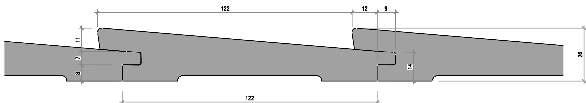
Nr. 7702-00-03 Stülpchalung N+K 14/26/122 mm, Rückseitig ausgekehlt
