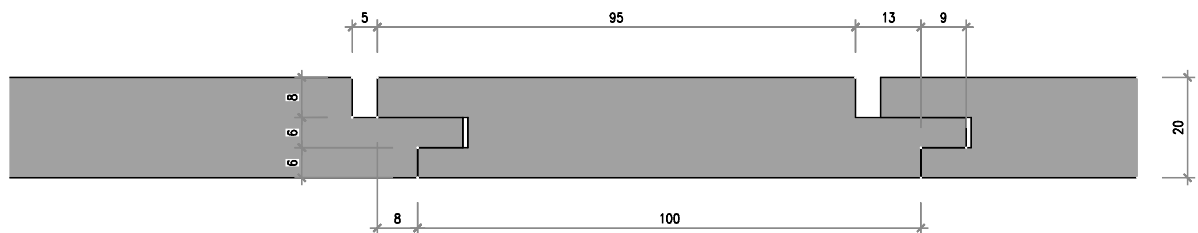
Nr. 2206-05-00 Sichtnutschalung gerade 20/100 mm, scharfkantig
