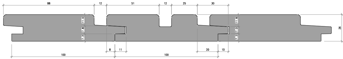
Nr. 2272-12-03 Sichtnut Trio gerade mit verschobener Mittelnut, 3 Teile
