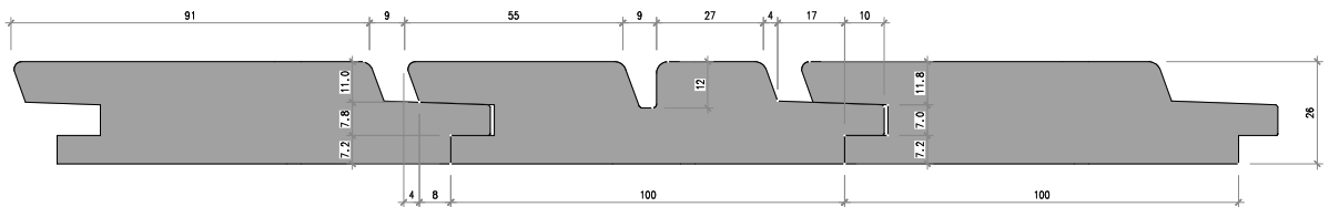
Rhomboid N+K Trio mit verschobener Mittelnut, Radius 3 mm, 3 Teile
