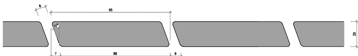
Nr. 6501-4k-03 Rhomboidschalung 20° 20/95 mm
