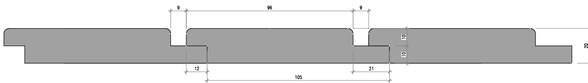
Nr. 8001-09-03 Wechselfalz mit Sichtnut gerade
