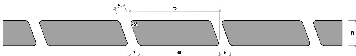
Nr. 6501-4k-03 Rhomboidschalung 20° 20/72 mm
