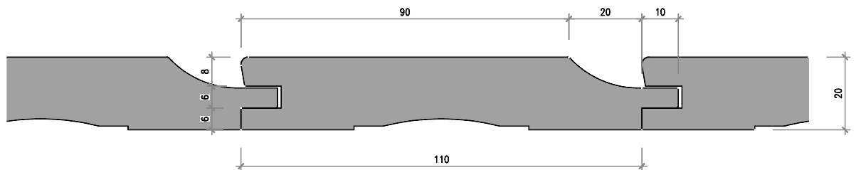
Nr. 7101-20-03 Chaletschalung 20/110 mm, ausgekehlt, Kante gerundet
