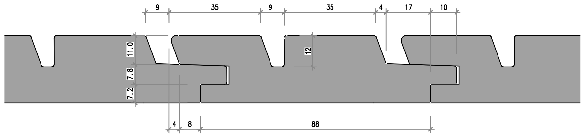
Nr. 6622-09-03 Rhomboid N+K 26/88 mm, mit Mittelnut
