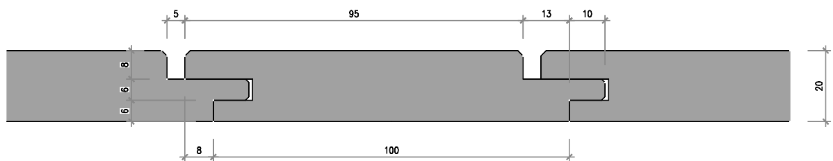
Nr. 2204-05-02 Sichtnutschalung gerade 20/100 mm, Fase 2 mm
