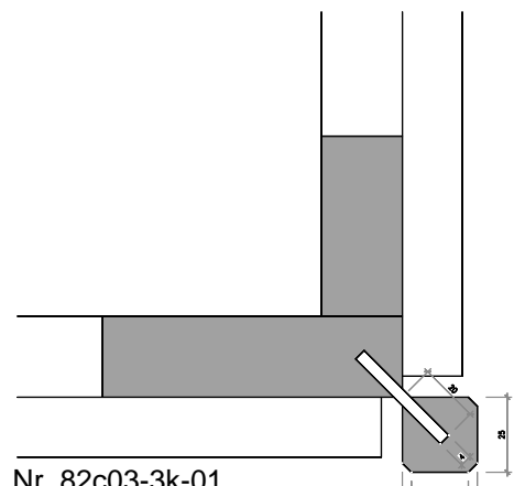
Nr. 82c03-3k-01 Fassadeneckprofil Smart 25/25 mm mit 4/20 mm Nut, Fase 3 mm
