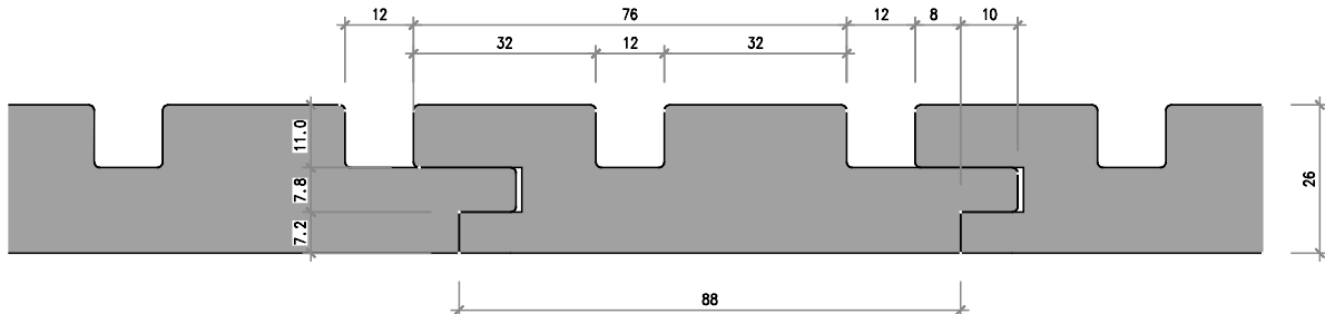
Nr. 2222-12-03 Sichtnutschalung gerade 26/88 mm mit Mittelnut, Kamm 10mm Für verdeckte Montage
