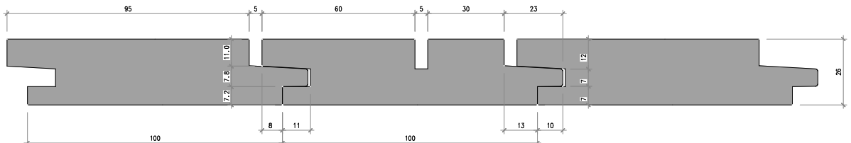
Nr. 2276-05-00 Sichtnut Trio gerade mit verschobener Mittelnut, 3 Teile
