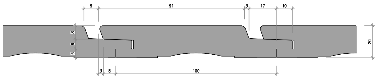
Rhomboidschalung N+K 20/100 mm
