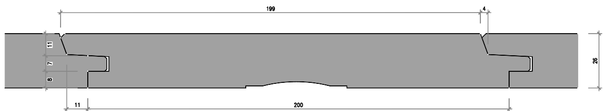
Nr. 6604-00-02 Strickwandimitation N+K 26/200 mm (Für nicht bewitterte Flächen)
