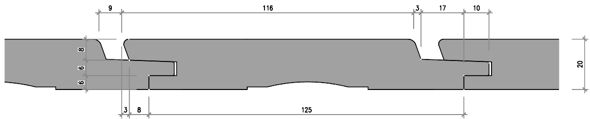
Rhomboidschalung N+K 20/125 mm
