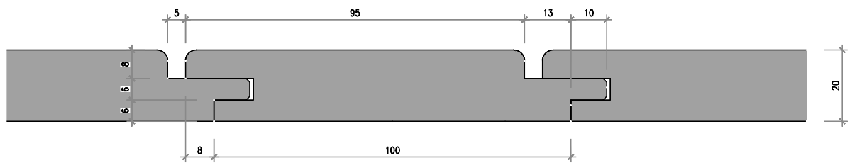
Nr. 2202-05-03 Sichtnutschalung gerade 20/100 mm, Nut 5 mm, Radius 3 mm
