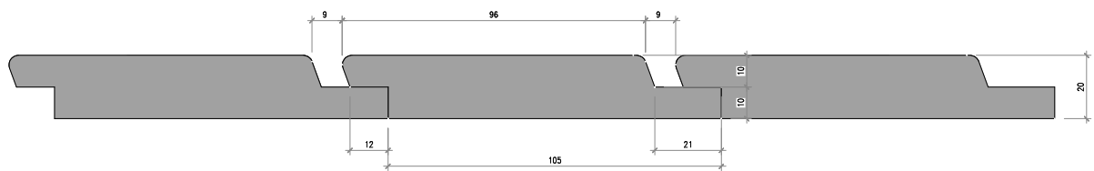
Nr. 6001-09-03 Wechselfalz mit Rhomboid 20°
