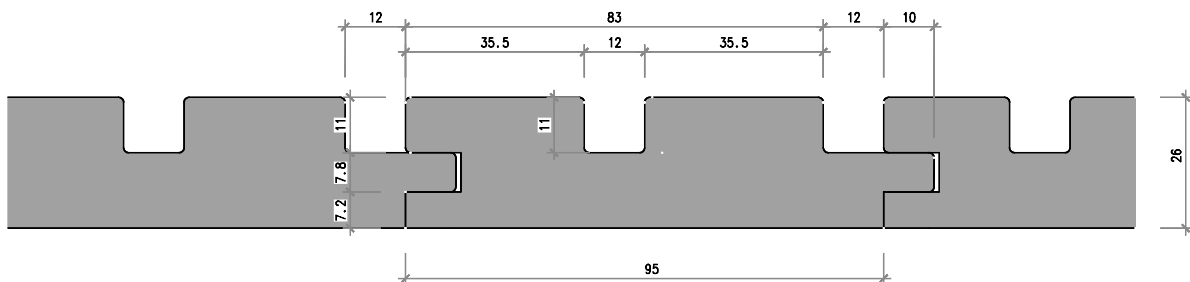
Nr. 2221-12-03 Sichtnutschalung gerade 26/95 mm mit Mittelnut, Kamm 10 mm
