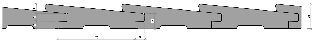
Nr. 7702-00-03 Stülpchalung N+K 14/23/70 mm, Rückseitig ausgekehlt
