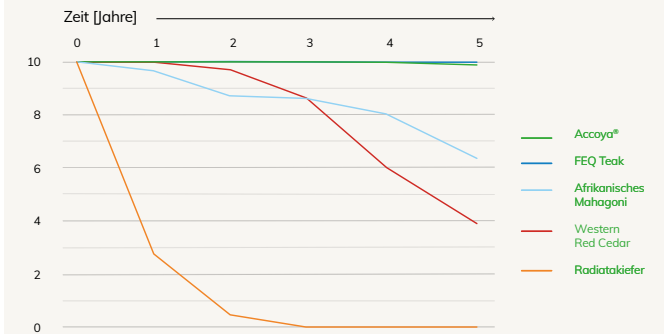
5-Jahres-Zerfallsrate (E18 Bodennähe)
