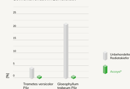
Gewichtsverlust im Zerfallstest
