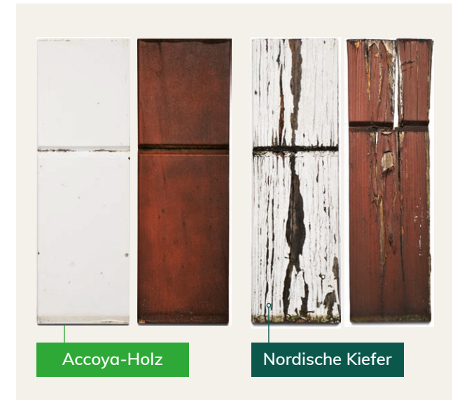
Vergleich externer Beschichtungen
