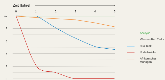
5-Jahre Termitentest (Gainesville FL, E18. Bodennähe)
