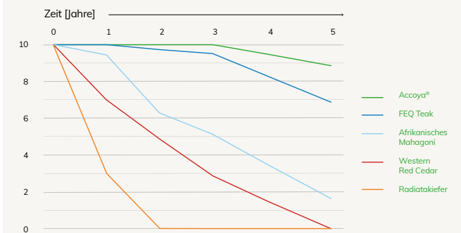
5 Jahre Zerfallsrate (E7 Bodenkontakt)
