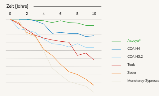
Zersetzungsdaten von Bodenpfählen [Zustandsindex]
