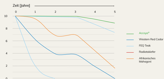
5-Jahre Termitentest (Gainesville FL, E7 Bodenkontakt)
