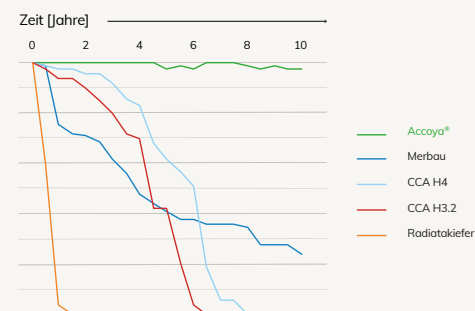
Zersetzungsdaten von Bodenpfählen [Zustandsindex]
