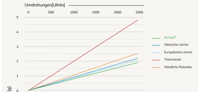
Gewichtsverlust durch Taber-Abrieb
